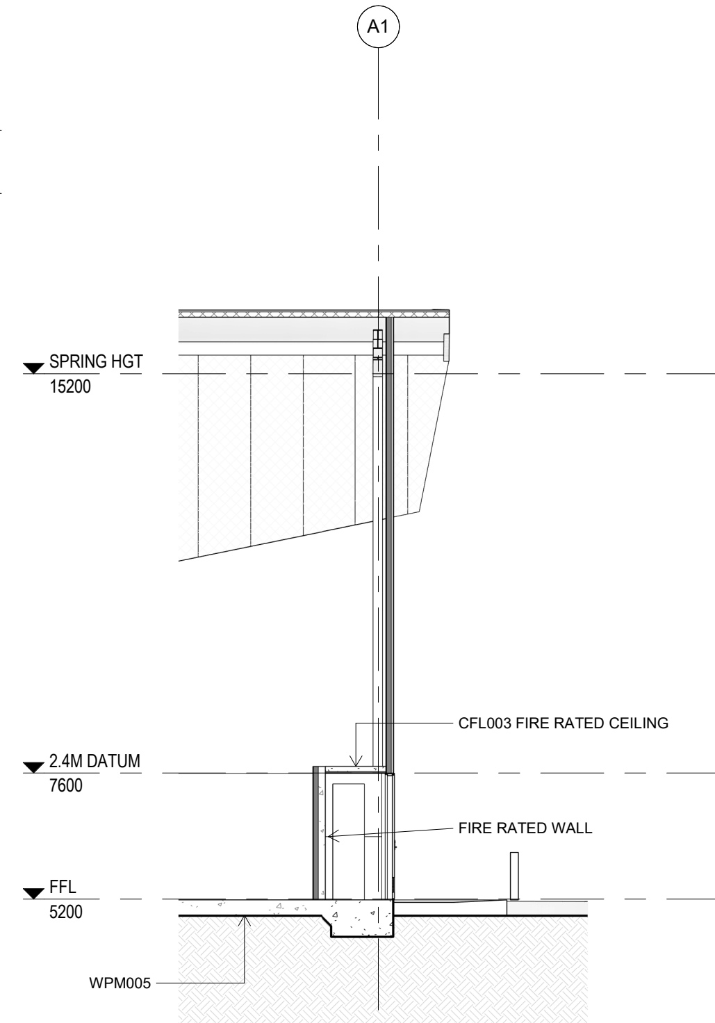
2 SECTION - GRIDS 3A 1 : 100
